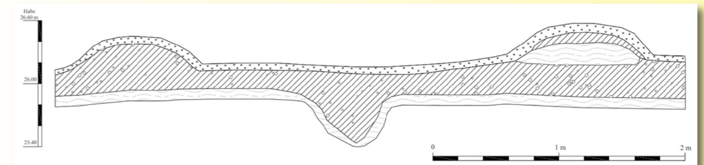
Pav. 3. Klaipėdos krašto sienos griovio tyrimai Bartinkų miške. perkasos Nr. 3 ŠŠR sienelėje fiksuotas kaip spėjama, buvusio patruliavimo kelio profilis. Brėžinio autorius A. Skrupskelis, parengta pagal M. Marcinkevičiūtės ataskaitos duomenis.
