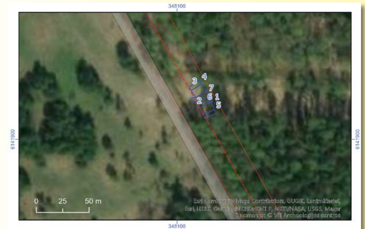
Pav. 2. Klaipėdos krašto sienos griovio tyrimai Bartinkų miške. Tyrimų vieta ir perkasų išdėstymas.
