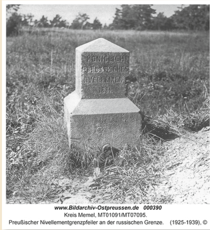
Pav. 1. Prūsijos karalystės niveliacinių matavimų kraštiniai reperiai. Kairėje – Lauksargių akmuo su niveliaciniu reperiu 7847. Reperis užpiltas gruntu. E. Mažrimo nuotrauka, 1981 m. (Mažrimas 2020, p. 854). Dešinėje – Analogiškas akmuo Nemirsetoje su niveliaciniu reperiu 7381. Niveljavimo reperis matosi ties žemės paviršium, žolėse. Iš www.Bildarchiv-Ostpreussen.de
