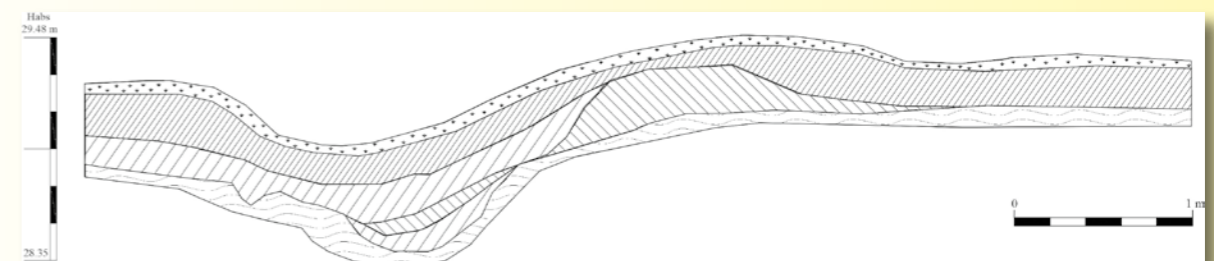
Pav. 6. Viršuje – 2014 m. tyrimų vieta Saulažolių k. pagal tyrimų vadovo M. Mačiulio ataskaitą. Apačioje – tyrimų perkastos sienelės brėžinys. Autorius – A. Skrupskelis, pagal M. Mačiulio ataskaitoje pateiktus duomenis.
