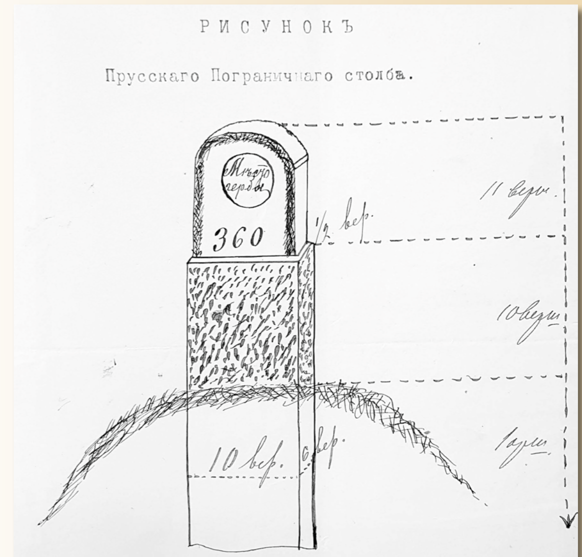
Pav. 7. Prūsijos sienos akmeninio žymeklio (stulpo) brėžinys. Matmenys duoti verškais ir aršinais. Ant stulpo pažymėtas Nr. 360 rodo, kad eskizas pieštas pagal netoli Kretingos buvusį sienos ženklą. Viršutinėje dalyje apskrityje užrašas „Herbo vieta“. Kauno regioninis valstybės archyvas. F. 473 Ap. 1. B. 4584 L. 132
