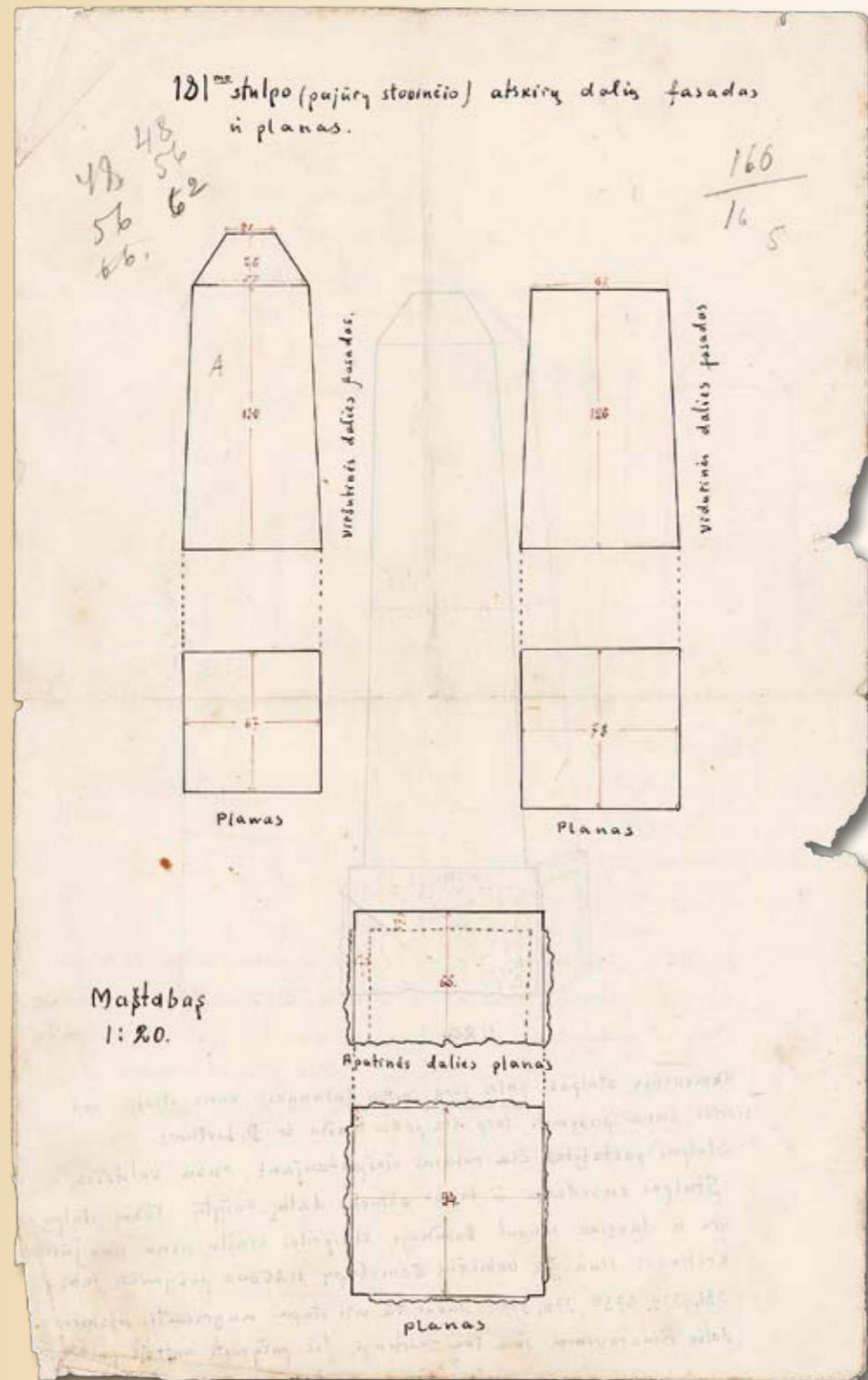
Pav. 15. Lietuvos kariuomenės majoro Juozo Šarakausko archyvinė medžiaga su Rusijos Imperijos pasienio akmeninių stulpų/obeliskų išmatavimais. Nacionalinio Mikalojaus Konstantino Čiurlionio dailės muziejaus fondai GP 57411
