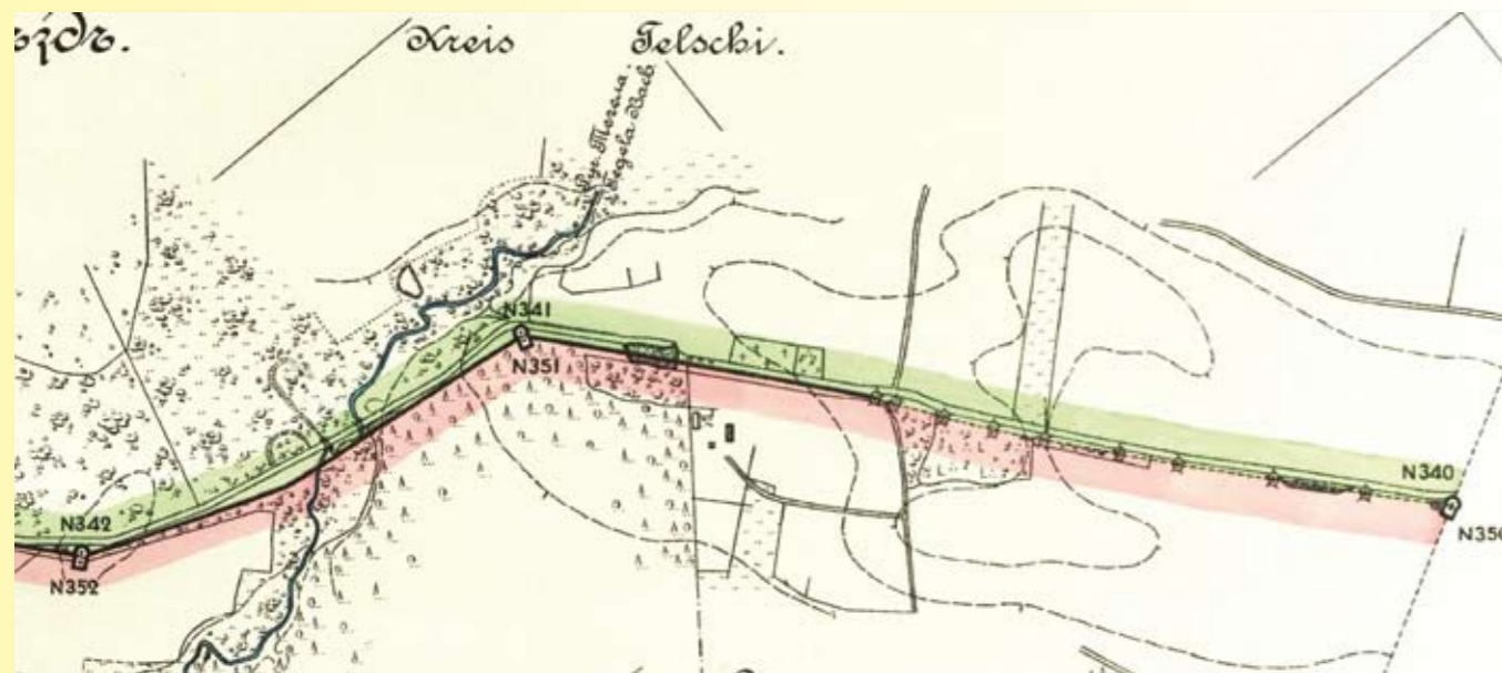
Pav. 5. 2012 m. tirta sienos vieta ant XIX a. pabaigos – XX a. pradžios sienos demarkavimo plano. Planas orientuotas į rytus, t.y. šiaurė yra į kairę.
